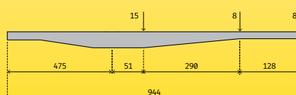
PS18X45D-HT-1500KG
